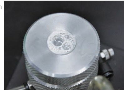
การทดสอบรอยรั่วโดยใช้ฟอง (JIS-Z2329)
