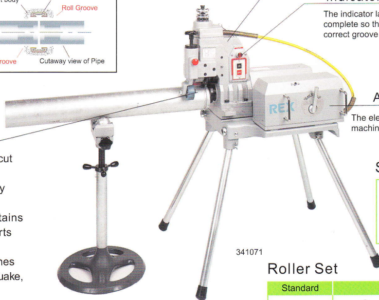
Roller
