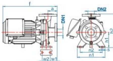
WCM-1505FS,FT/ WCM-2205FS,FT
