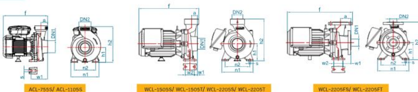
ACL-755S/ ACL-1105S
