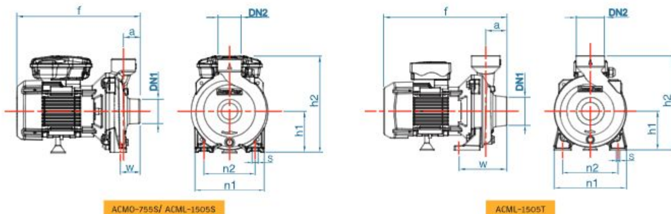
ACMO-755S/ ACML-1505S
