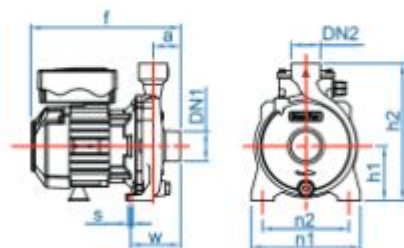
ACH-375S
