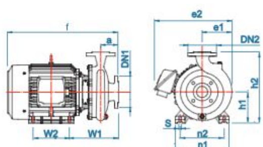
WCL-11005FT/ 15005FT
